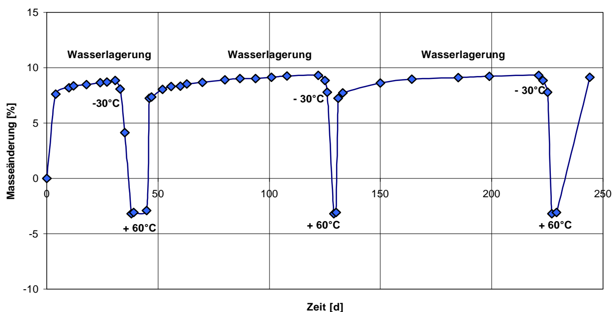
Abb. 2: Masseänderung infolge Aufnahme und Abgabe von Wasser; Durchschnittswert von drei gelgetränkten Ziegelproben
